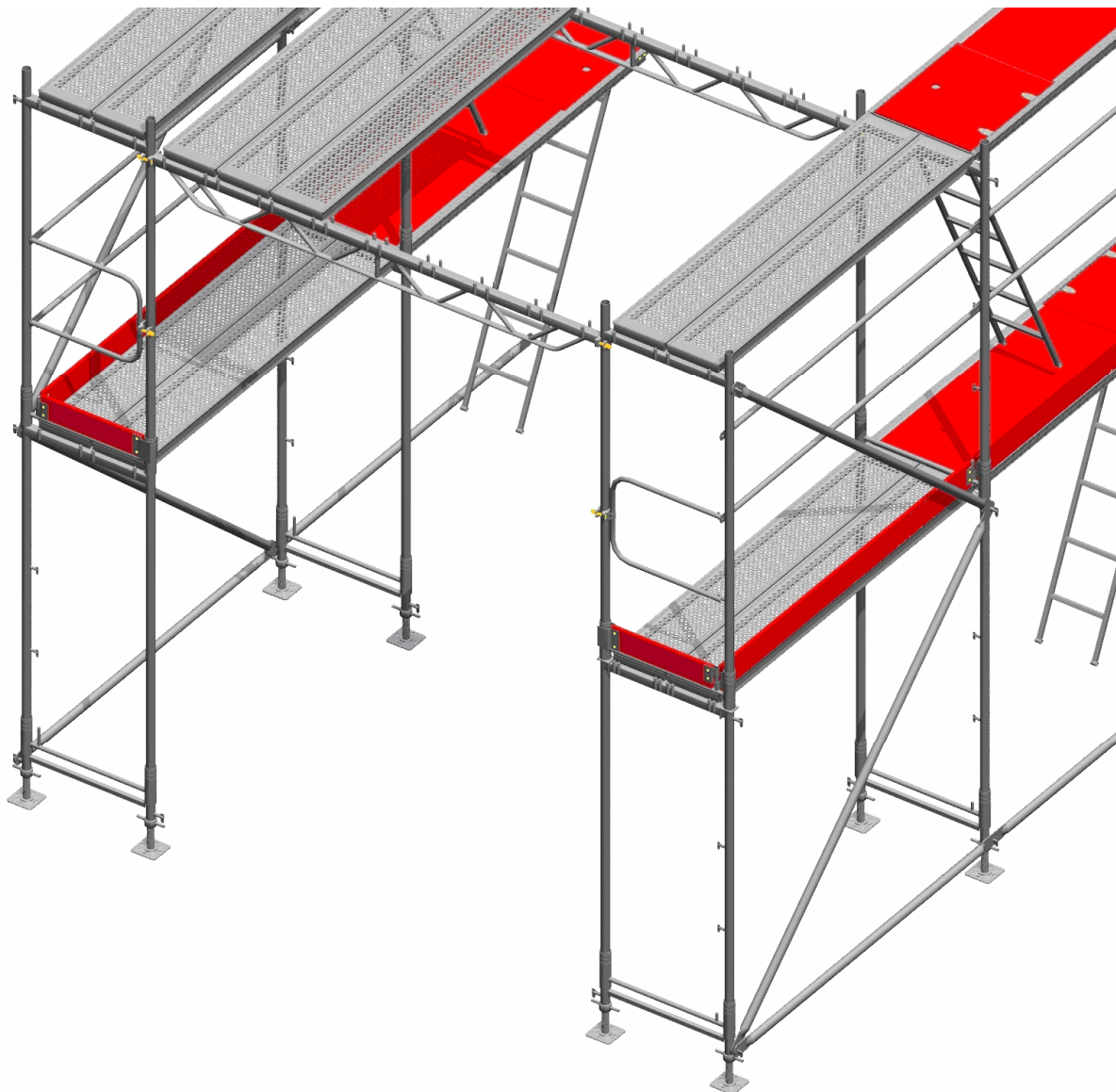
Rys. 1. Zastosowanie trawersów
